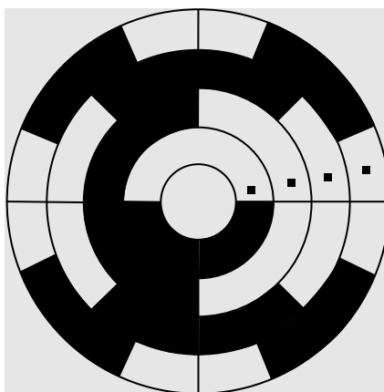
Рис. 13.2. Датчик углового положения
