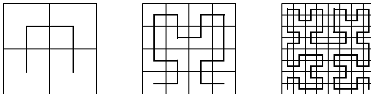
Рис. 14.1. Первые три кривые в последовательности, определяющей кривую Гильберта
