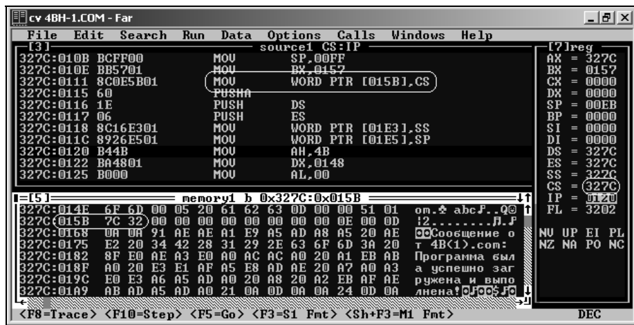
Рис. 29.3. Готовим EPB
