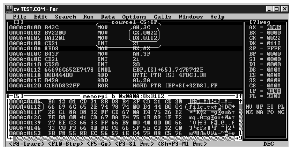
Рис. 19.1. Создание файла
