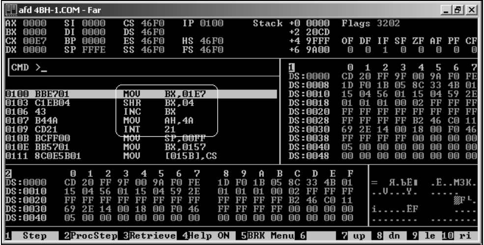
Рис. 29.1. Урезаем память
