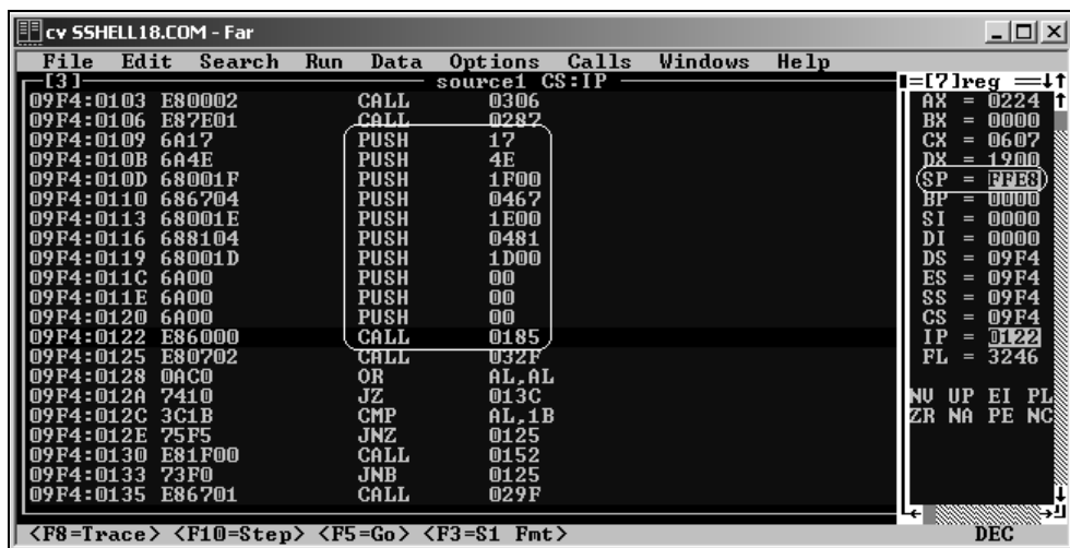
Рис. 18.1. Передача параметров в стеке
