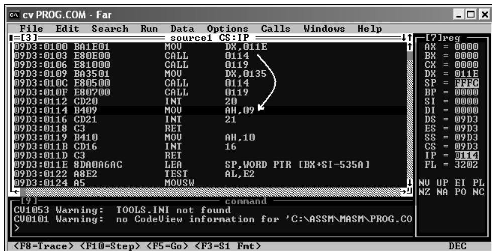
Рис. 5.1. Вызов подпрограммы
