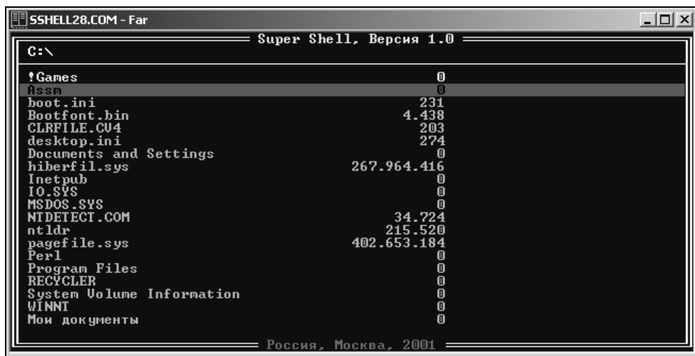
Рис. 28.4. Выделение файла
