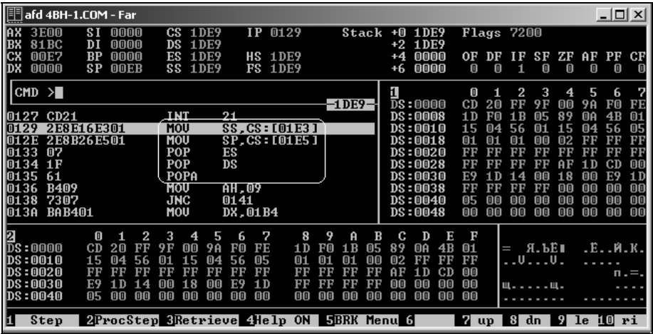
Рис. 29.6. Восстановление регистров
