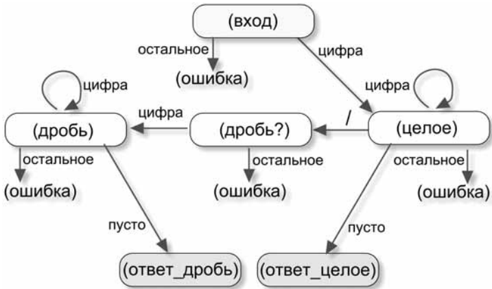
Рис. 17.2. Диаграмма переходов
