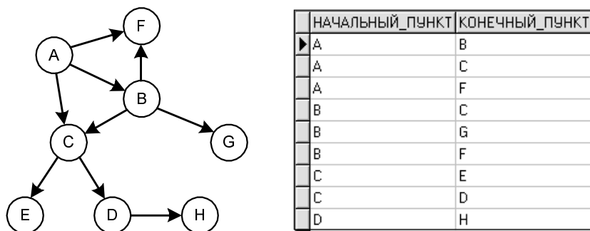
Рис. 5.4. Граф и таблица достижимости пунктов
