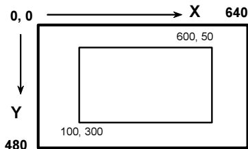
Рис. 1.6. Прямоугольник со сторонами, параллельными экрану
