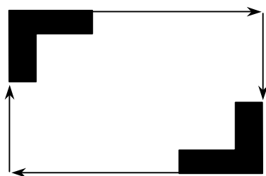
Рис. 1.71. Две змейки
