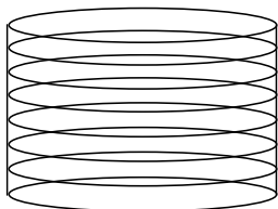
Рис. 1.16. Цилиндр
