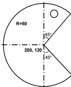
Рис. 1.20. CD-MAN
