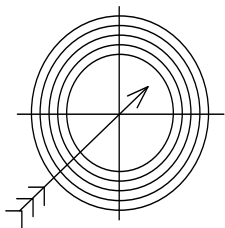
Рис. 1.14. Мишень
