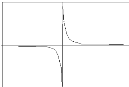
Рис. 1.48. График гиперболы
