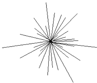
Рис. 1.46. Взрыв
