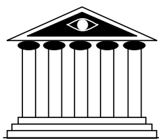
Рис. 1.27. Храм
