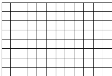
Рис. 1.36. Решетка
