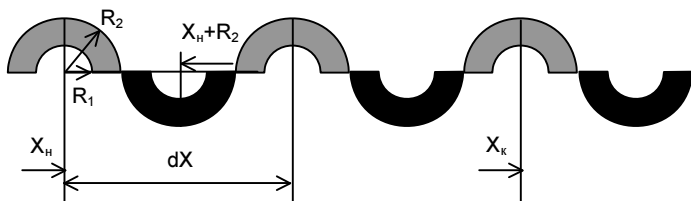
Рис. 1.40. Орнамент
