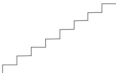
Рис. 1.54. Лестница 2
