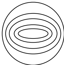
Рис. 1.57. "Эллипсирующие окружности"
