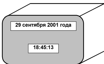
Рис. 1.61. Электронный будильник
