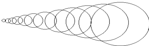
Рис. 1.49. "Рупор"
