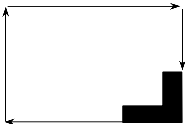
Рис. 1.70. Сторож-змейка
