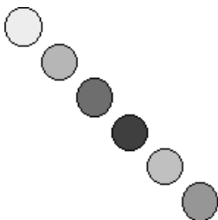
Рис. 1.64. Разноцветные круги
