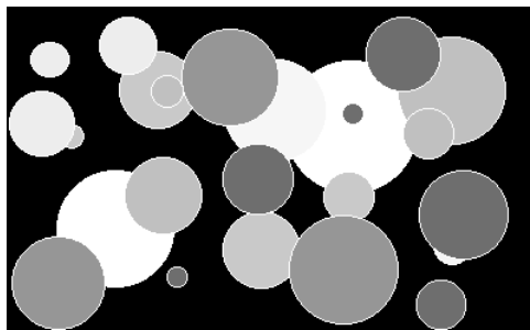
Рис. 1.45. Разноцветные окружности
