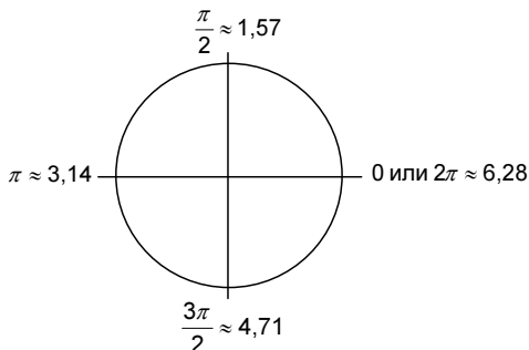
Рис. 1.18. Тригонометрическая окружность
