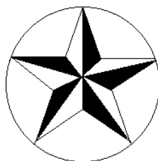
Рис. 1.25. Звезда
