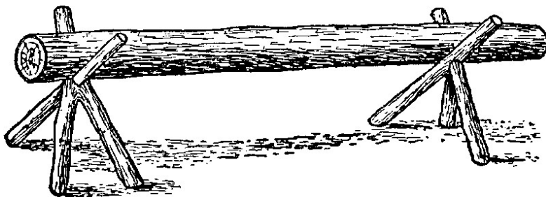
Рис. 2.12. Простые козлы
