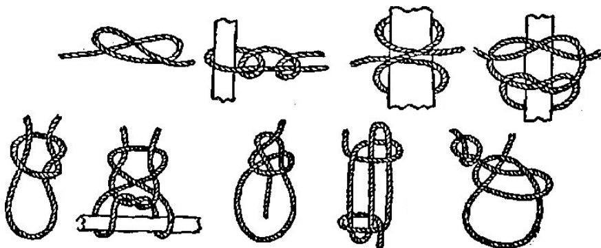
Рис. 4.20. Различные варианты «хитрых» деревенских узлов
