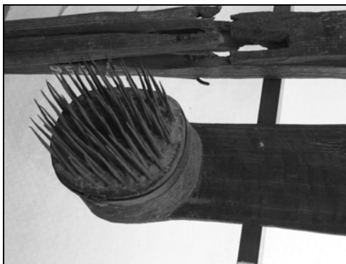
Рис. 4.10. Устройство для вычески пуха
