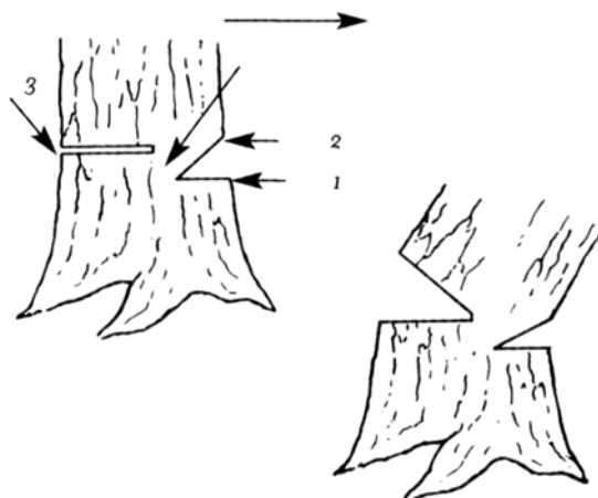
Рис. 2.11. Надрезы для спиливания большого дерева
