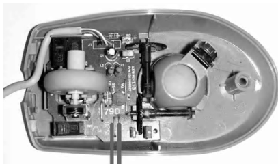
Рис. 3.14. Механическая компьютерная мышка со снятым корпусом: вид на печатную плату и механизм позиционирования координат
