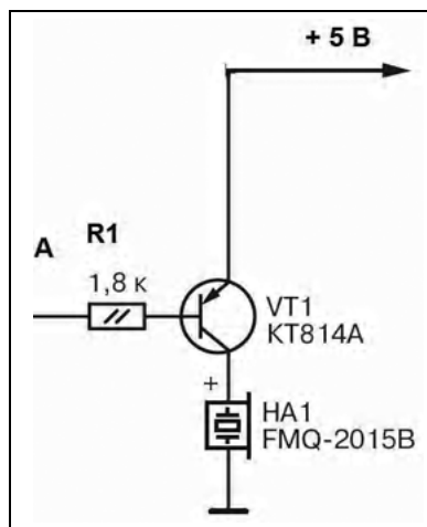
Рис. 3.16. Вариант схемы звукового сигнализатора для подключения к датчику смещения предмета (компьютерная мышь)
