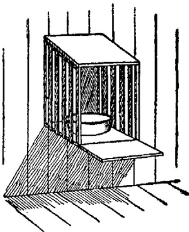
Рис. 4.15. Поилка для скотины, защищенная с боков
