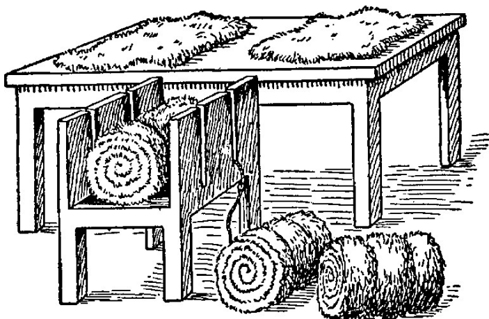
Рис. 4.11. Приспособление для сворачивания шкур в рулоны
