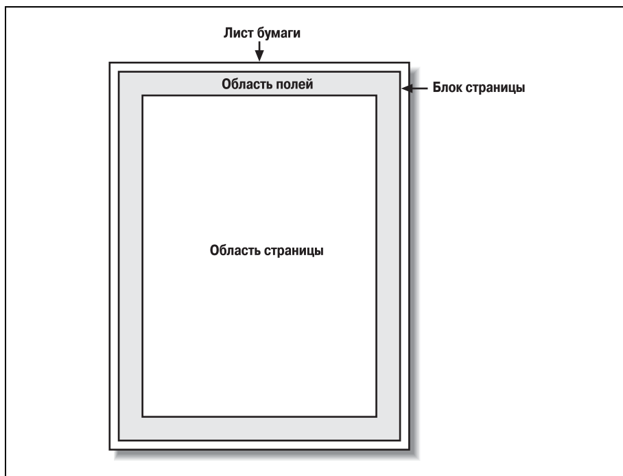
Рис. 14.1. Блок страницы
