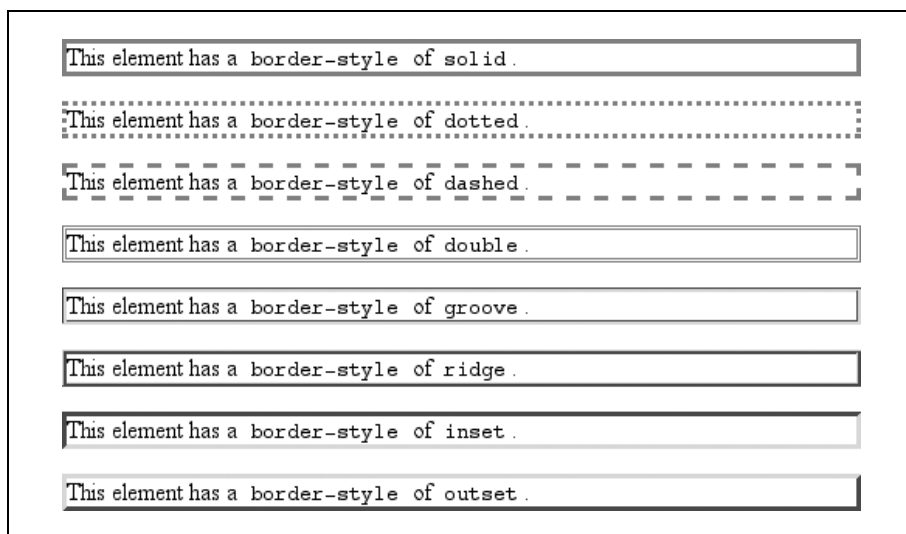
Рис. 8.20. Стили рамок
