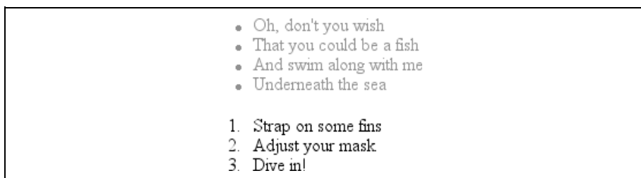
Рис. 3.3. Наследование стилей
