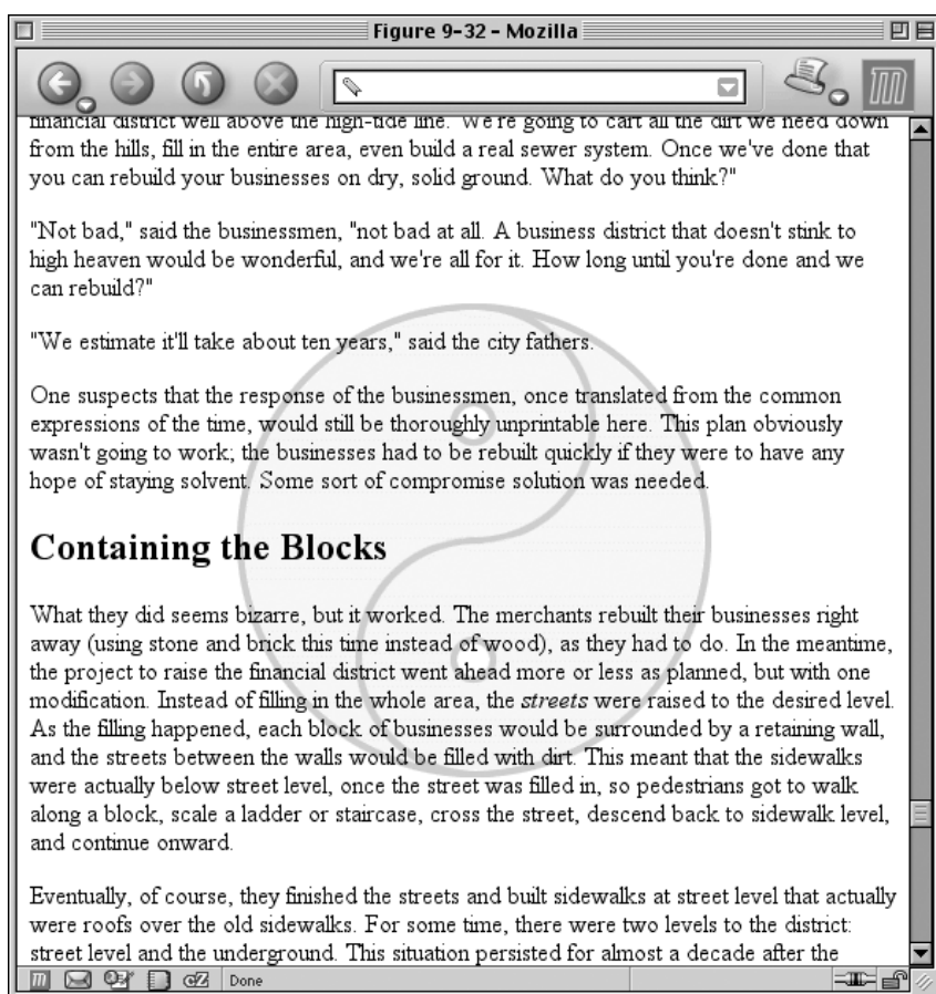
Рис. 9.32. Закрепление фона
