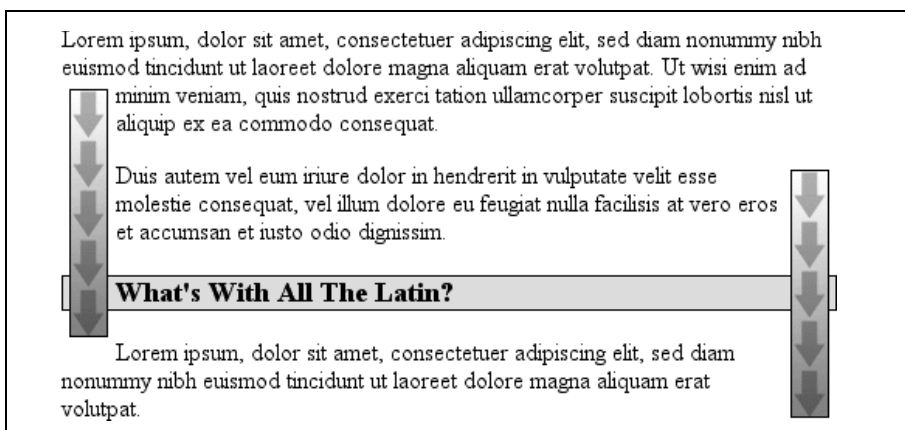
Рис. 10.24. Полностью обтекаемый
