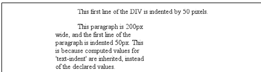
Рис. 6.4. Унаследованный отступ
