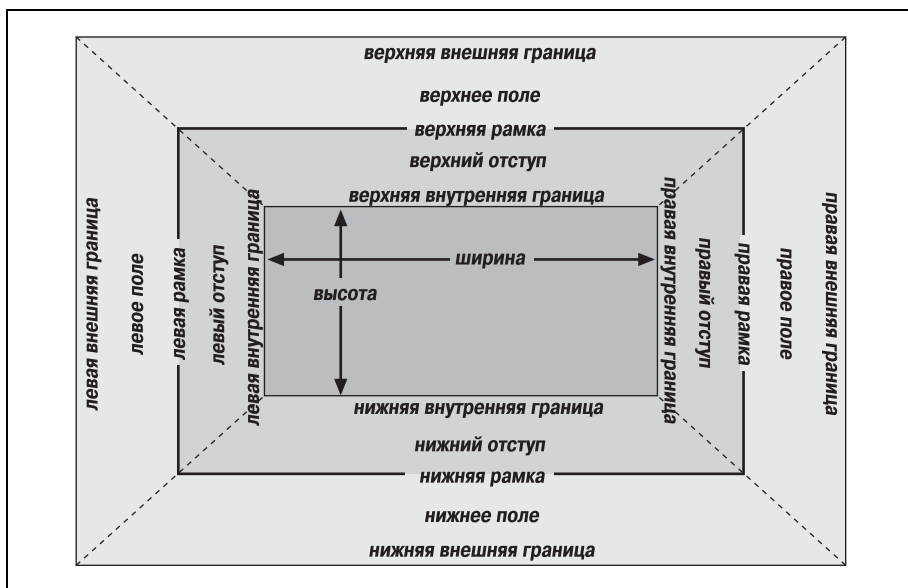
Рис. 7.2. Модель блока
