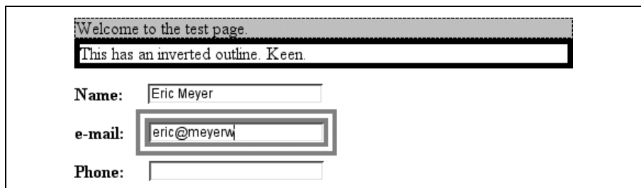
Рис. 13.14. Разные контуры
