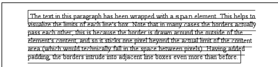
Рис. 7.41. Отступы и рамки не меняют высоту строки
