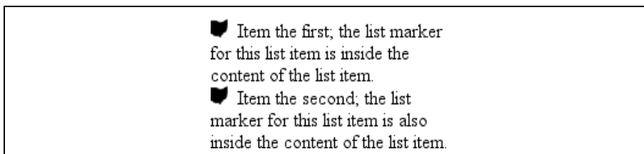
Рис. 12.6. Все вместе
