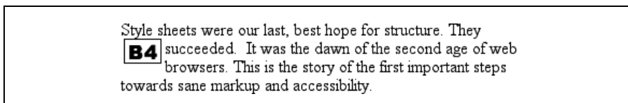
Рис. 10.1. Перемещаемое изображение
