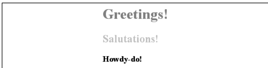
Рис. 4.1. Именованные цвета
