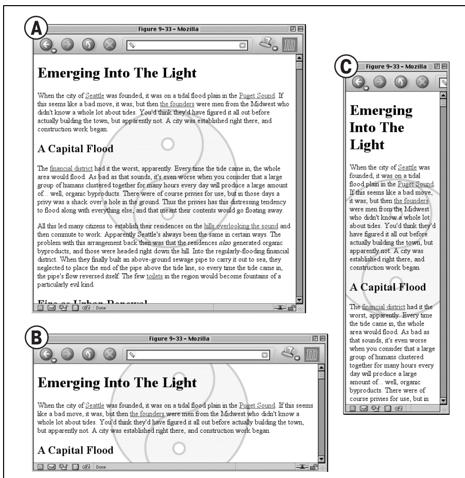
Рис. 9.33. Сохранение центрирования
