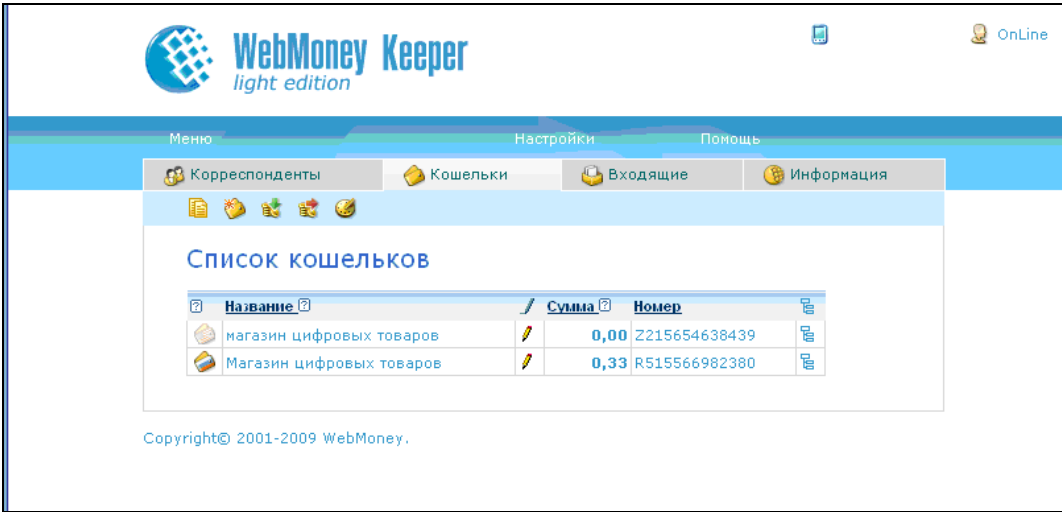
Рис. 3.27. Список кошельков
