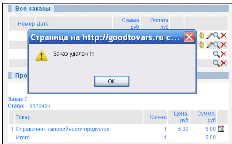
Рис. 3.46. Удаление заказа
