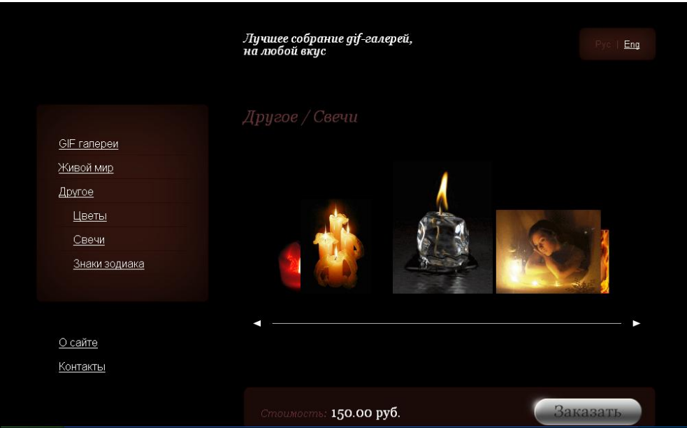
Рис. 1.33. Выбран пример 2_7
