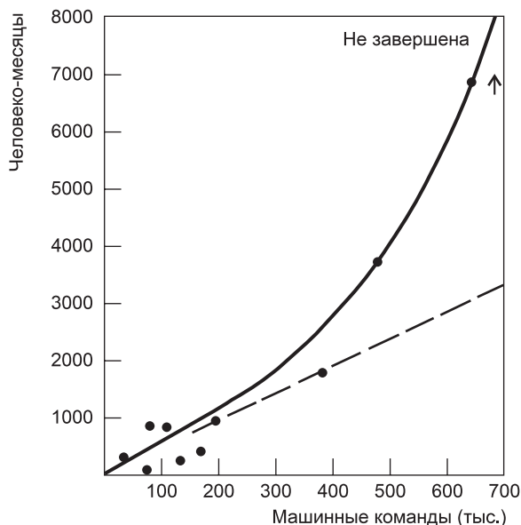
Рис. 8.1. Затраты на программирование как функция размера программы
