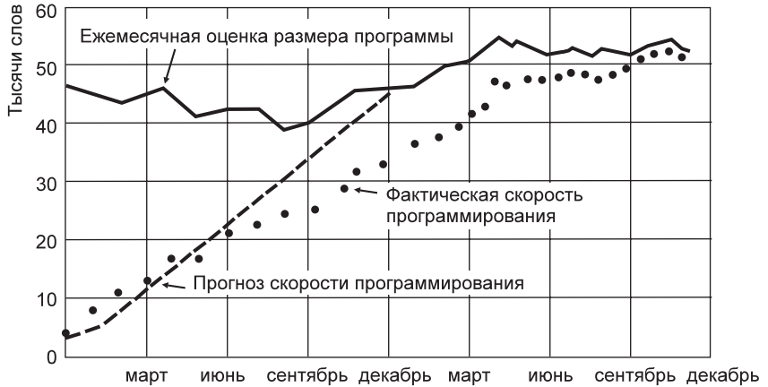
Рис. 8.3. Предсказанная и фактическая скорость программирования
