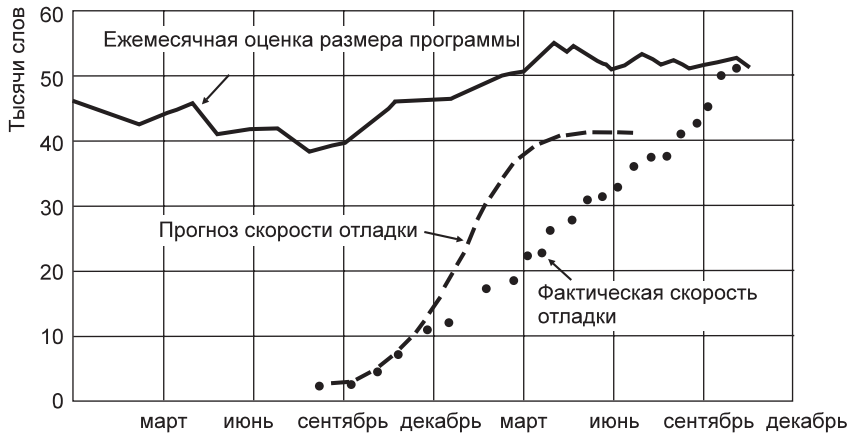
Рис. 8.4. Предсказанная и фактическая скорость отладки
