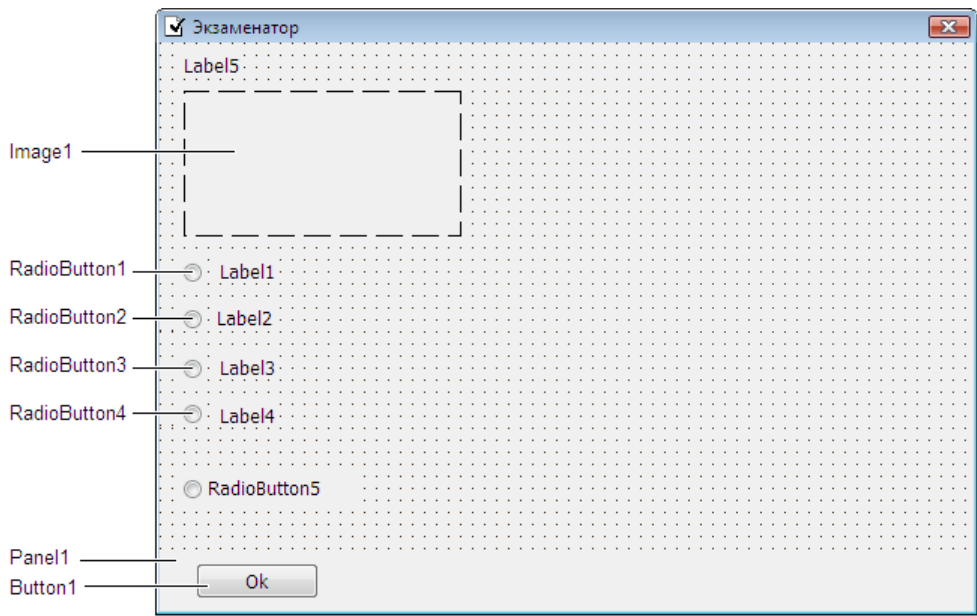
Рис. 10.2. Форма программы "Экзаменатор"
