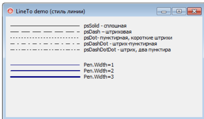
Рис. 4.4. Вид линии определяет значение свойства Pen.Style
