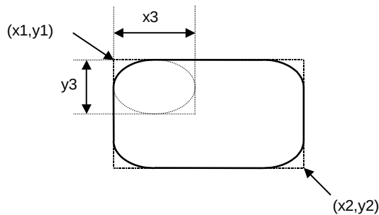
Рис. 4.8. Метод RoundRect вычерчивает прямоугольник со скругленными углами
