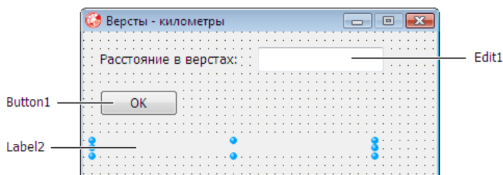
Рис. 3.6. Форма программы "Версты—километры"
