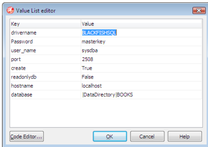
Рис. 6.24. Параметры соединения с БД Blackfish SQL Server
