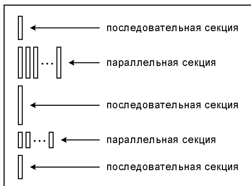
Рис. 5.2. OpenMP: процесс исполнения программы
