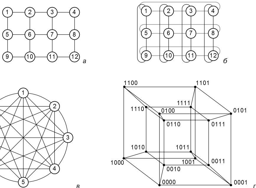
Рис. 2.14. Варианты топологий связи процессоров: а — решетка; б — 2-тор; в — полная связь; г — гиперкуб
