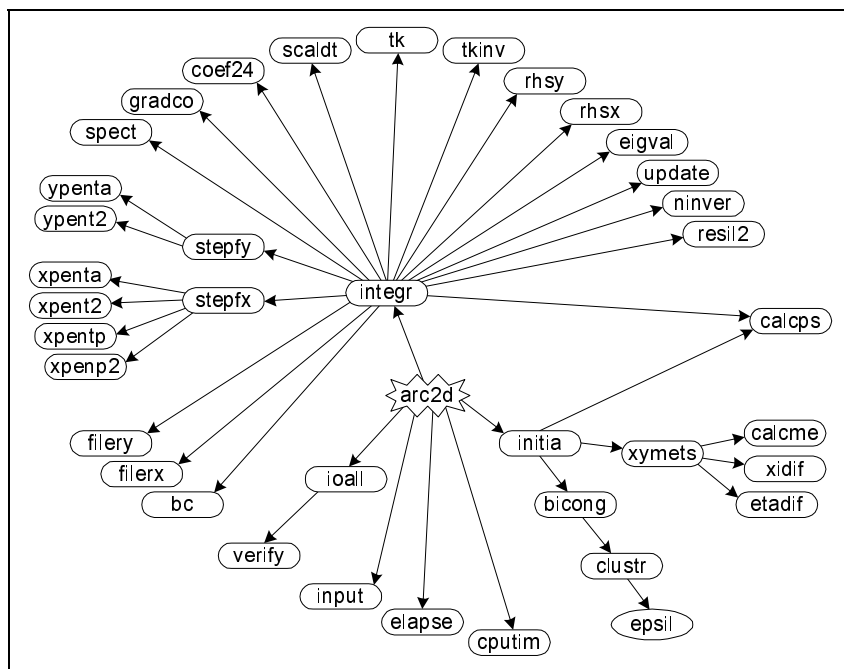
Рис. 9.5. Три варианта изображения одного и того же графа вызовов процедур ( окончание )
