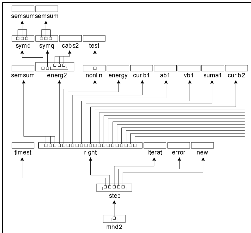
Рис. 9.6. Расширенный граф вызовов процедур
