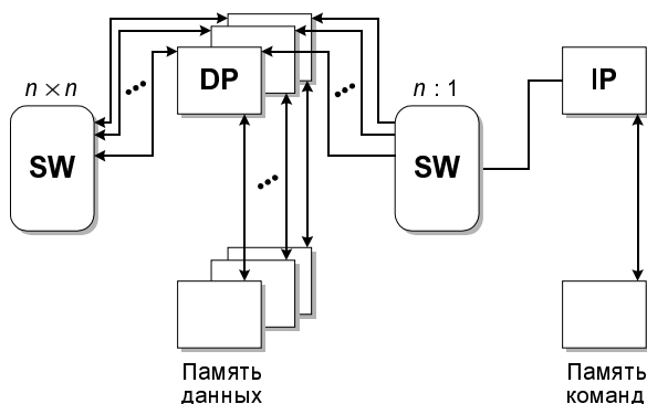
Рис. 3.6. Архитектура Connection Machine 2 в классификации Д. Скилликорна
