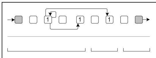
Рис. 9.11. Информационный граф
