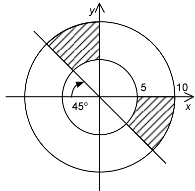
Рис. 8.5. Иллюстрация графической области к листингу 8.15
