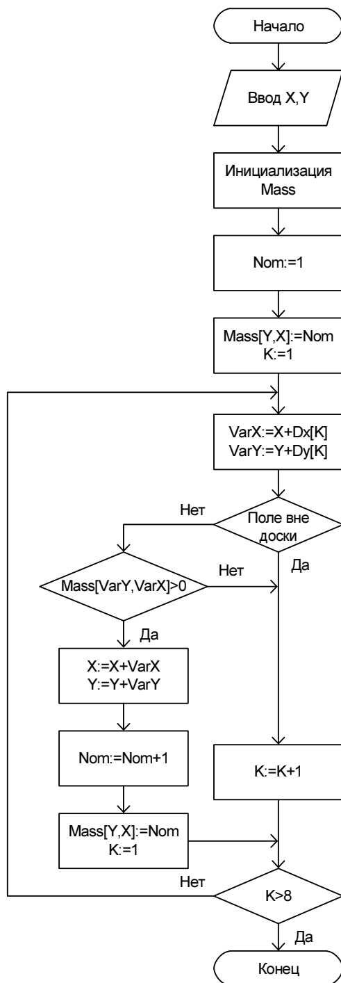
Рис. 4.4. Блок-схема к программе листинга 4.20
