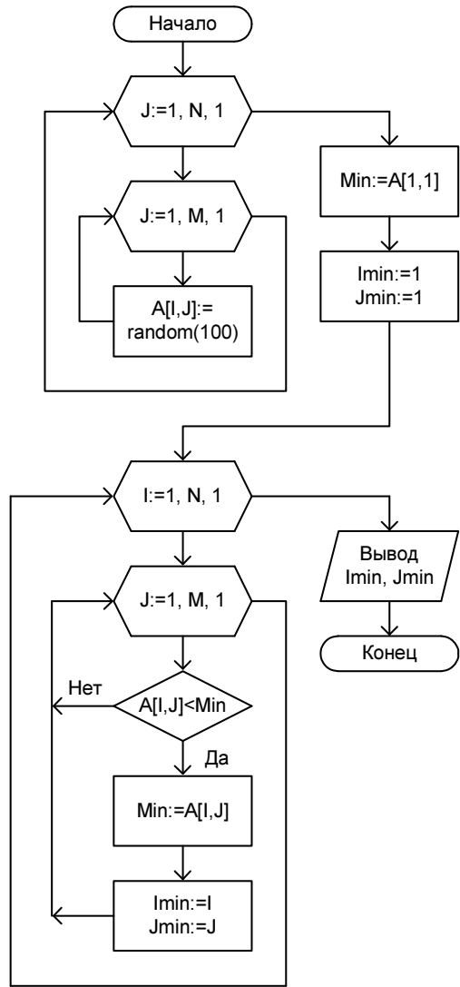
Рис. 4.1. Блок-схема к программе листинга 4.4
