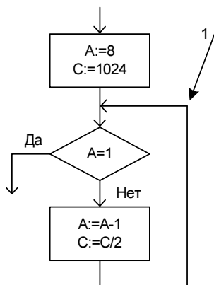
Рис. 2.26. Фрагмент алгоритма к задаче 2.11
