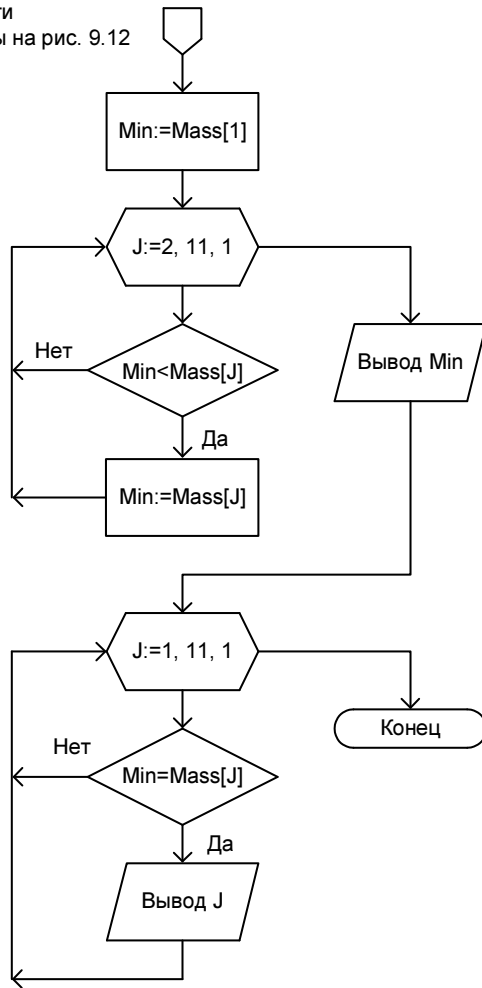
Рис. 9.13. Блок-схема (2 часть) к программе листинга 9.13
