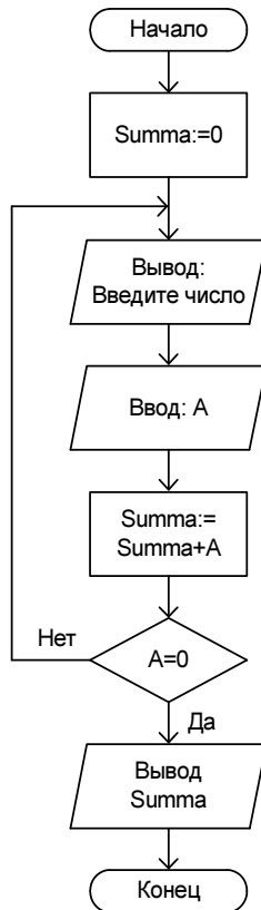
Рис. 2.14. Блок-схема к программе листинга 2.17
