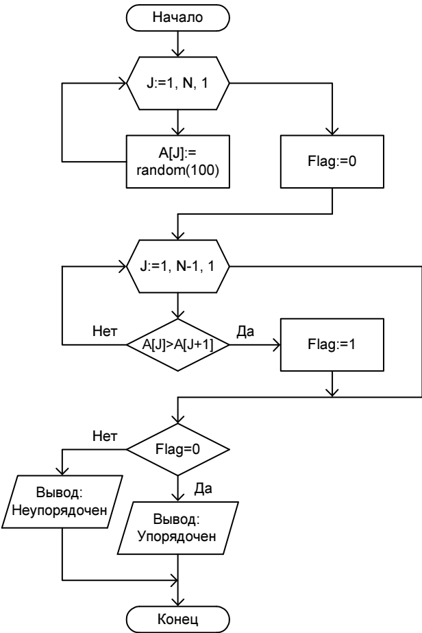
Рис. 3.3. Блок-схема к программе листинга 3.7
