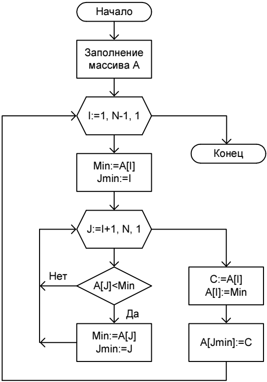
Рис. 9.11. Блок-схема к программе листинга 9.11
