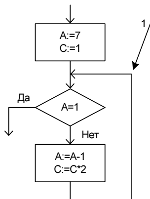
Рис. 2.25. Фрагмент алгоритма к задаче 2.10
