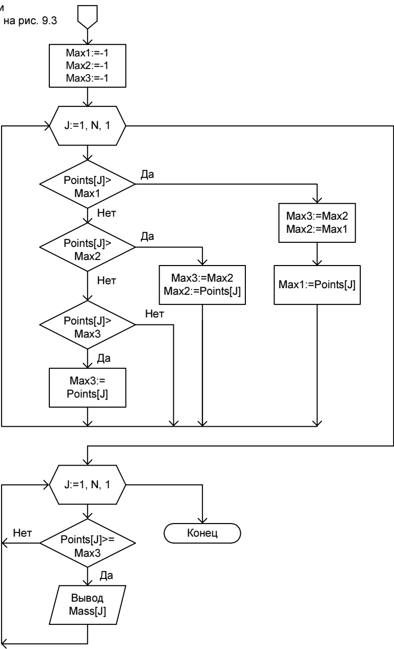
Рис. 9.4. Блок-схема (2 часть) к программе листинга 9.4
