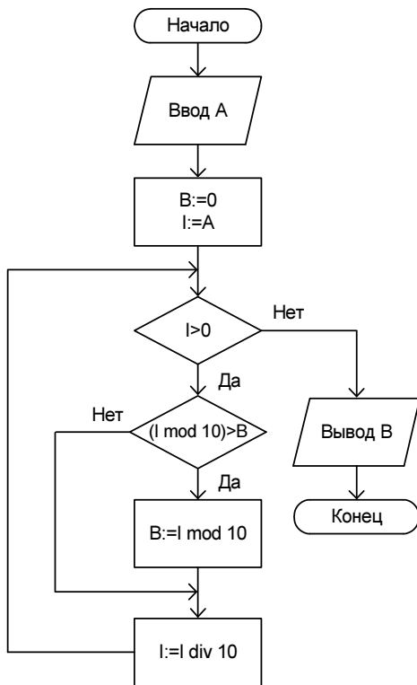
Рис. 2.22. Блок-схема к программе листинга 2.37
