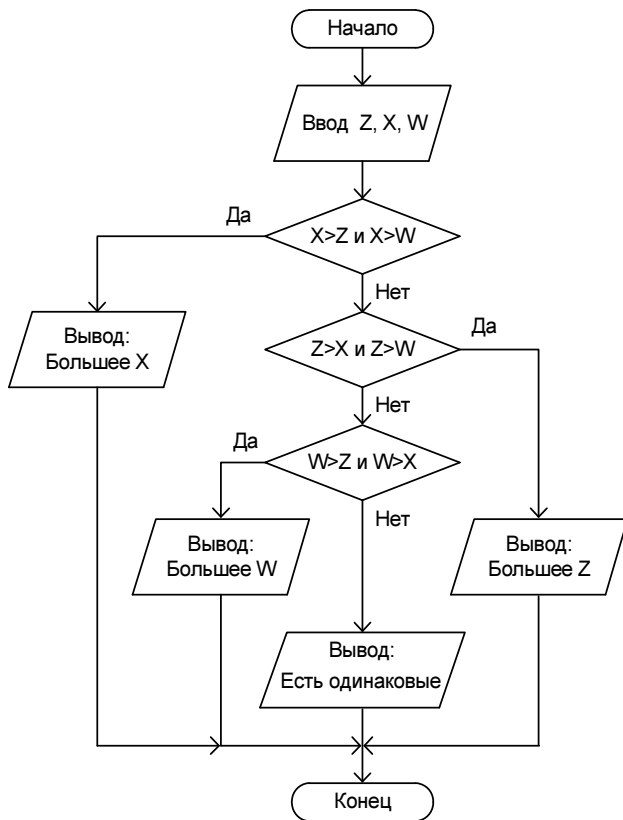
Рис. 2.4. Блок-схема к программе листинга 2.5
