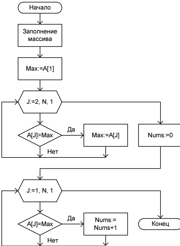
Рис. 3.8. Блок-схема к программе листинга 3.12
