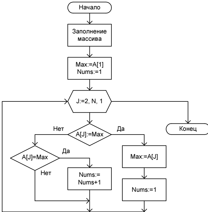
Рис. 3.9. Блок-схема к программе листинга 3.13
