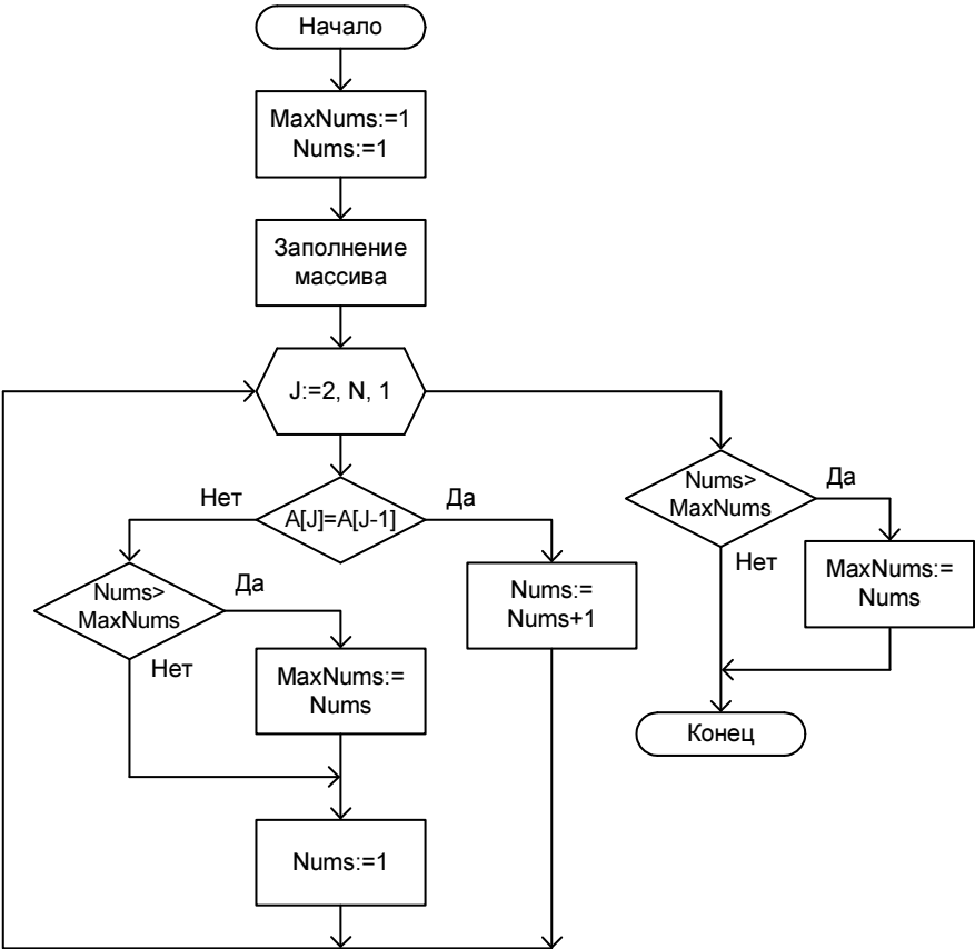
Рис. 3.7. Блок-схема к программе листинга 3.10
