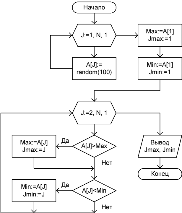
Рис. 3.2. Блок-схема к программе листинга 3.6
