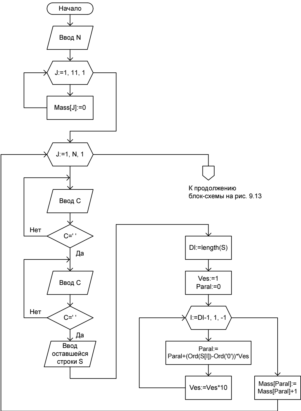
Рис. 9.12. Блок-схема (1 часть) к программе листинга 9.13
