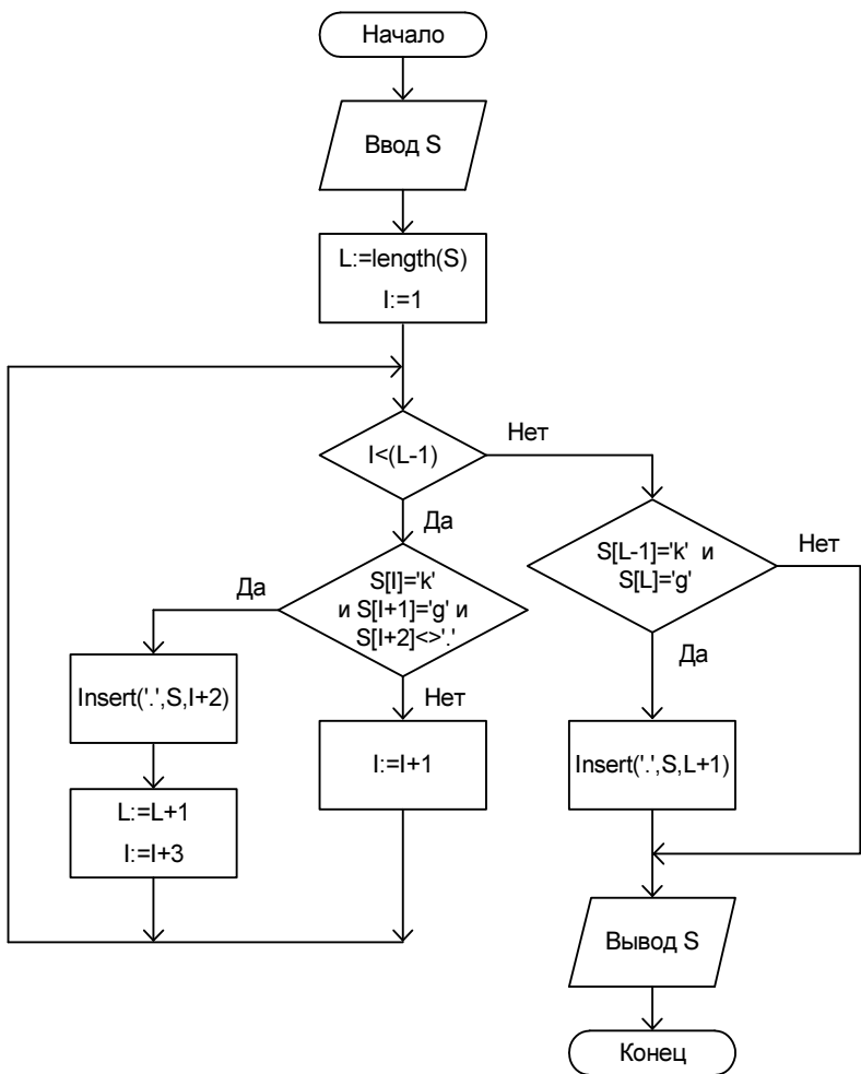
Рис. 5.2. Блок-схема к программе листинга 5.8
