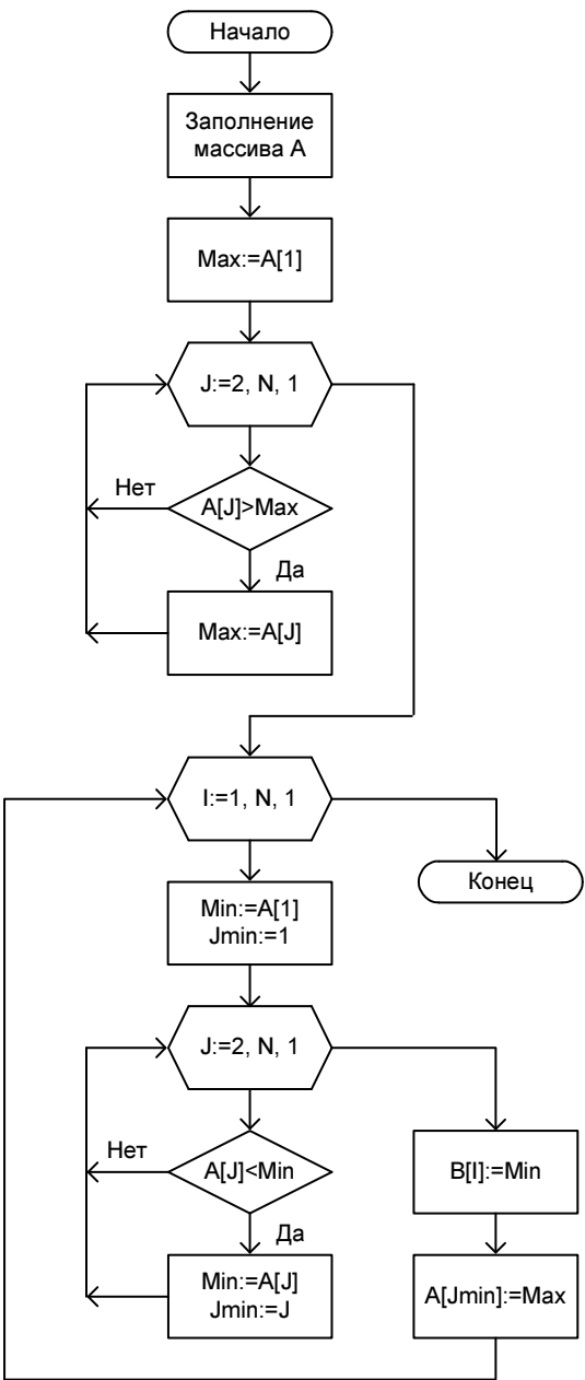
Рис. 9.10. Блок-схема к программе листинга 9.10
