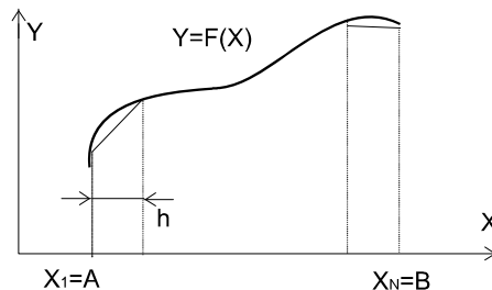
Рис. 8.3. График функции формулы (8.2) с разбивкой на трапеции
