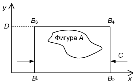
Рис. 8.8. Сложная фигура для вычисления площади
