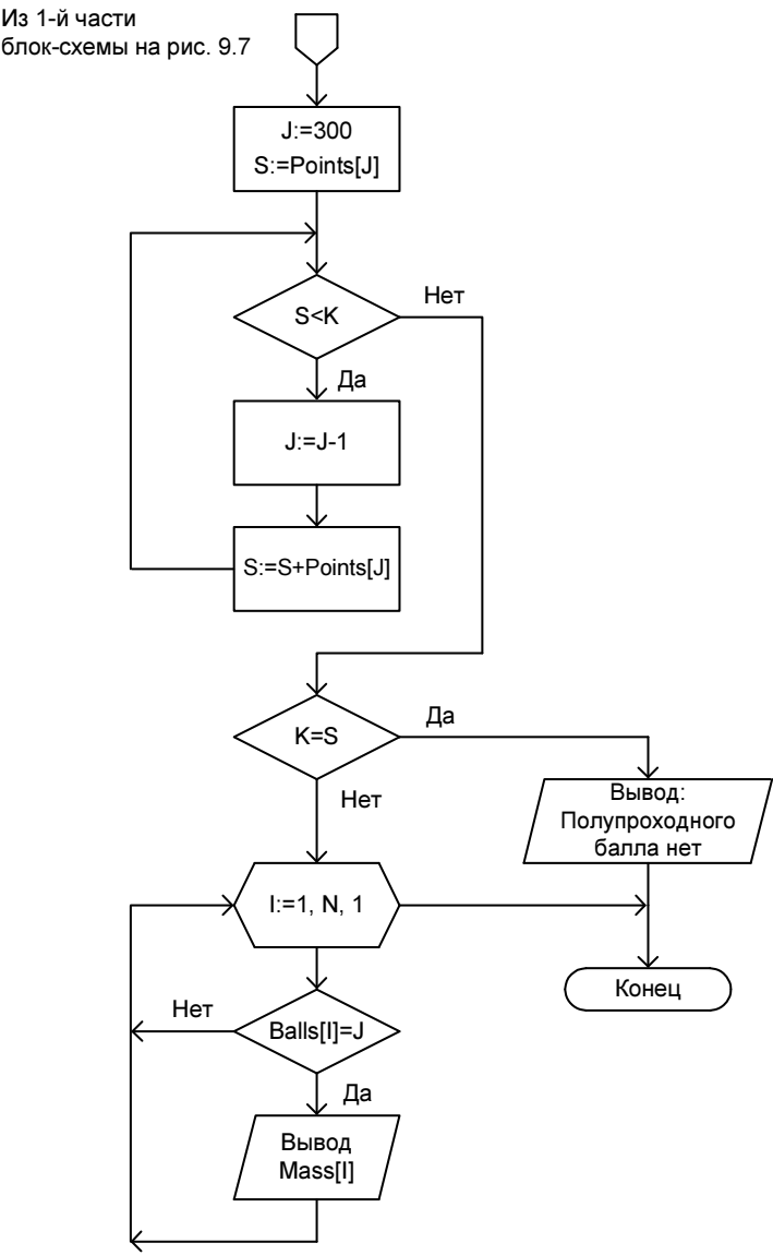
Рис. 9.8. Блок-схема (2 часть) к программе листинга 9.8
