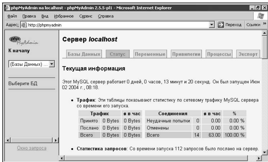
Рис 2.36. Страница состояния MySQL
