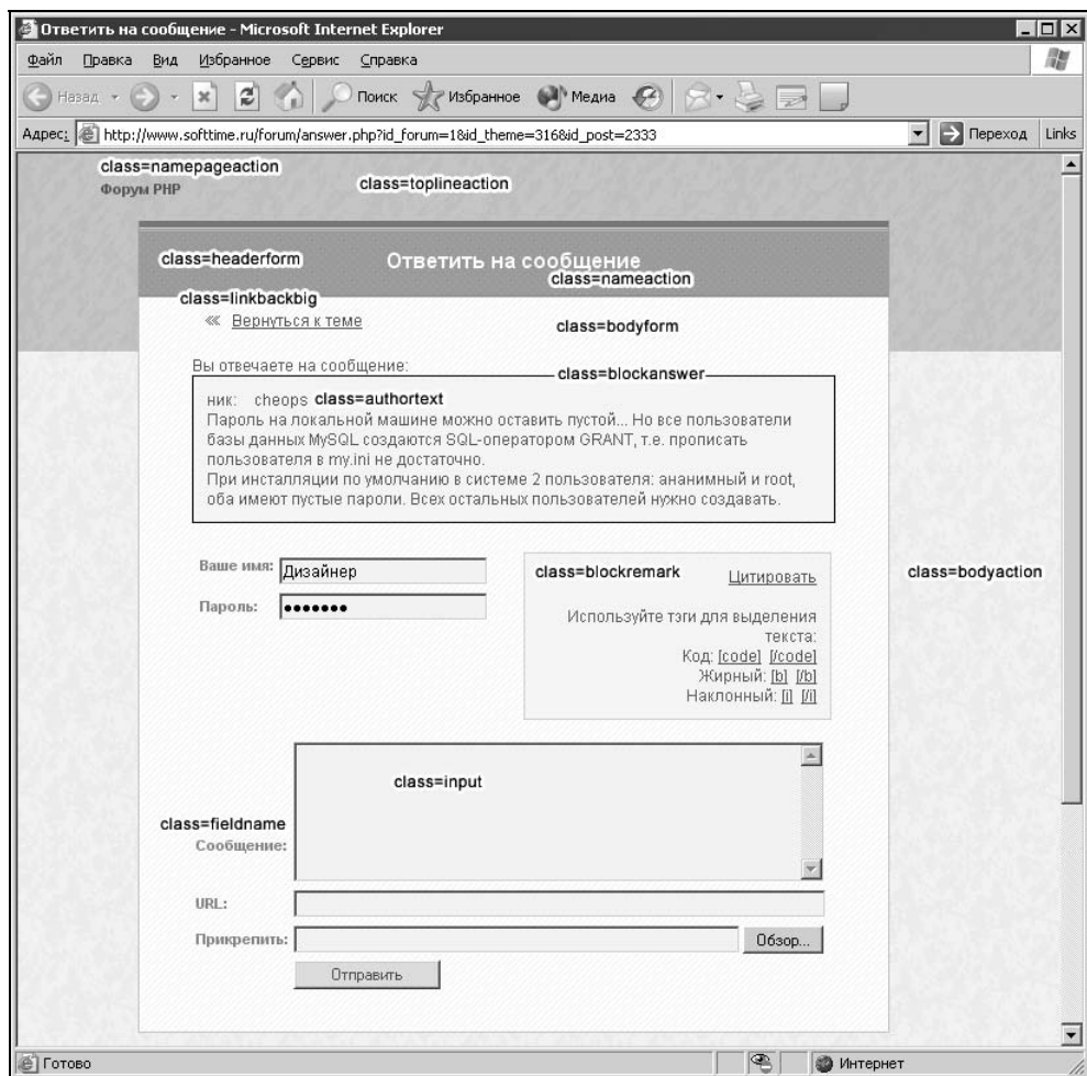
Рис. 20.12. Карта стилей для страницы answer.php
