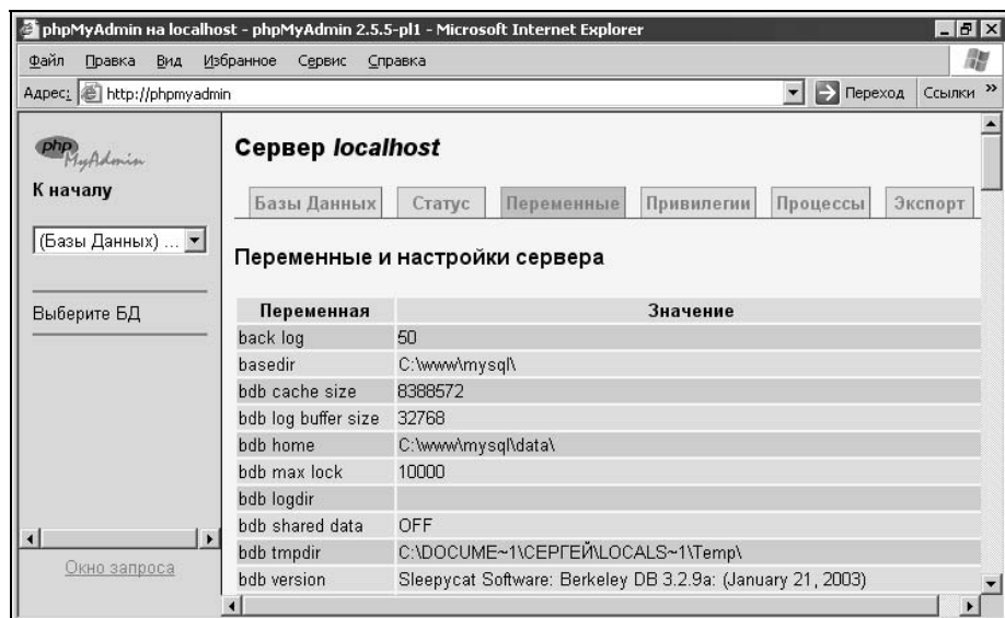
Рис. 2.37. Страница со списком системных переменных сервера MySQL
