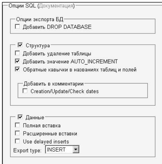
Рис. 2.43. Опции экспорта в формате SQL
