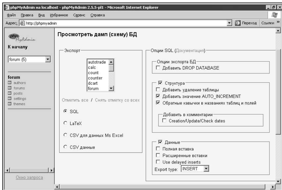
Рис. 2.41. Страница экспорта баз данных
