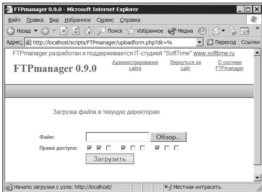
Рис. 16.3. Форма для загрузки файла на сервер
