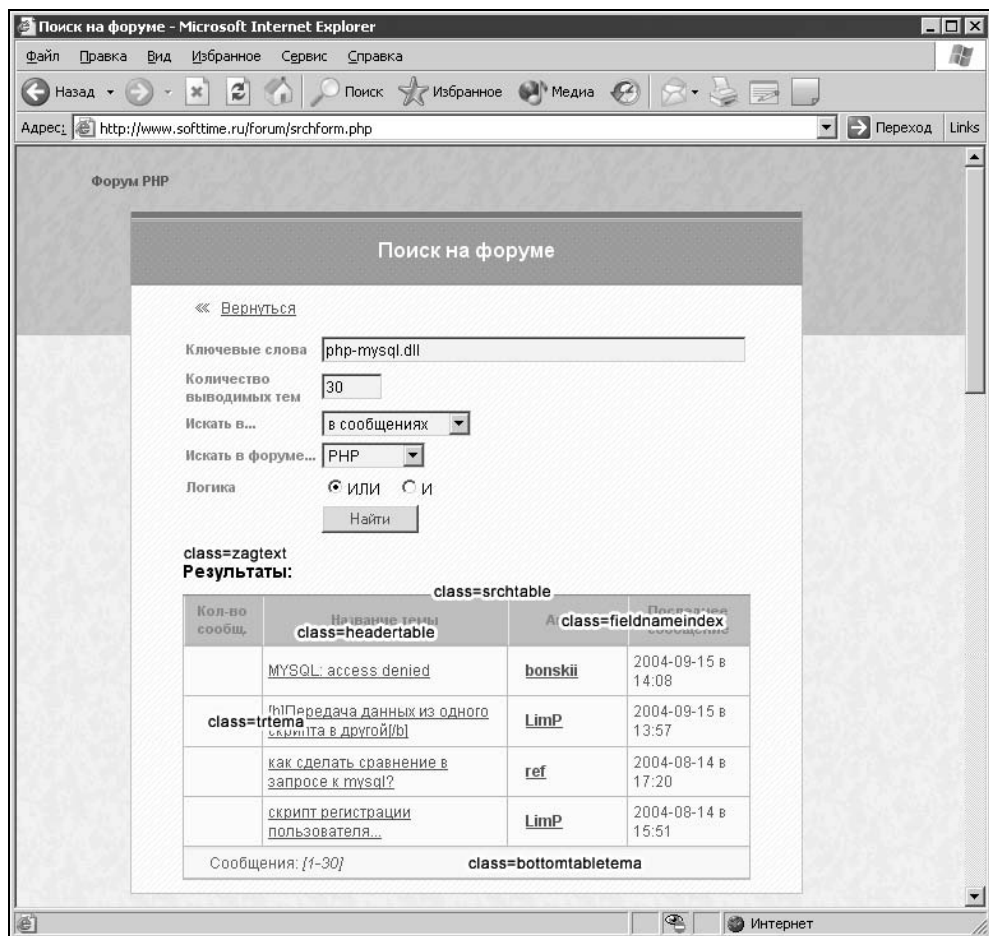
Рис. 20.13. Карта стилей для файла srchform.php
