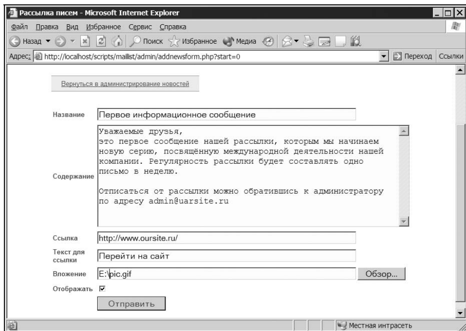
Рис. 18.2. Страница добавления новостной позиции
