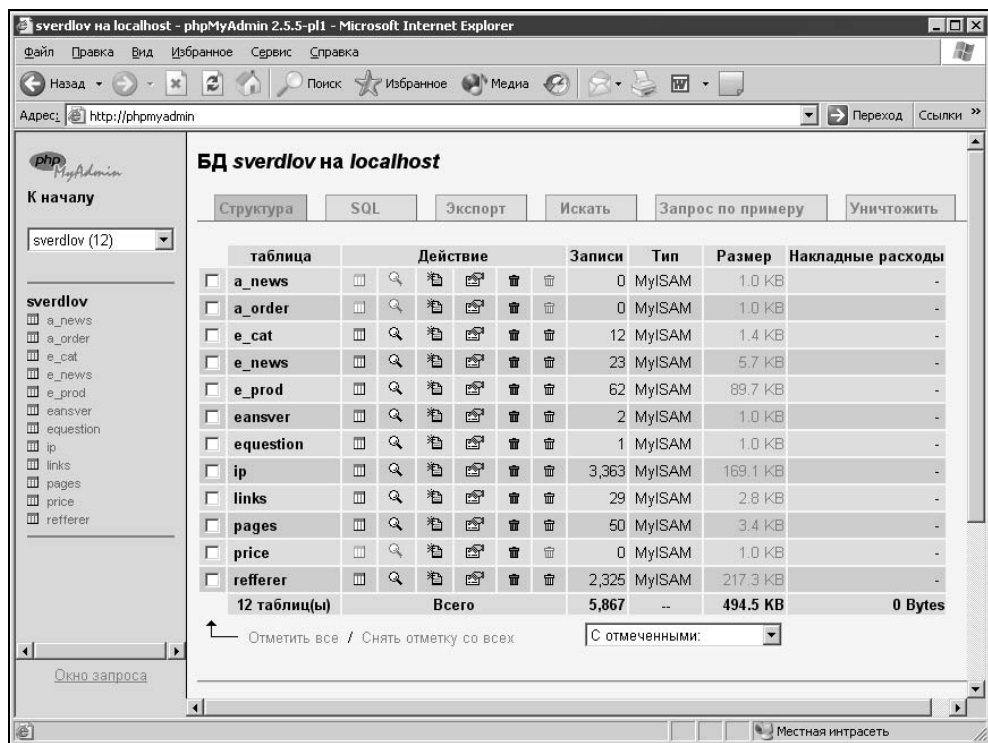
Рис 2.33. Интерфейс phpMyAdmin при работе с базой данных
