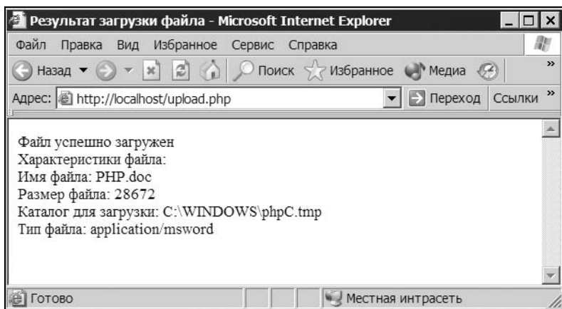
Рис. 4.2. Информация о загруженном файле
