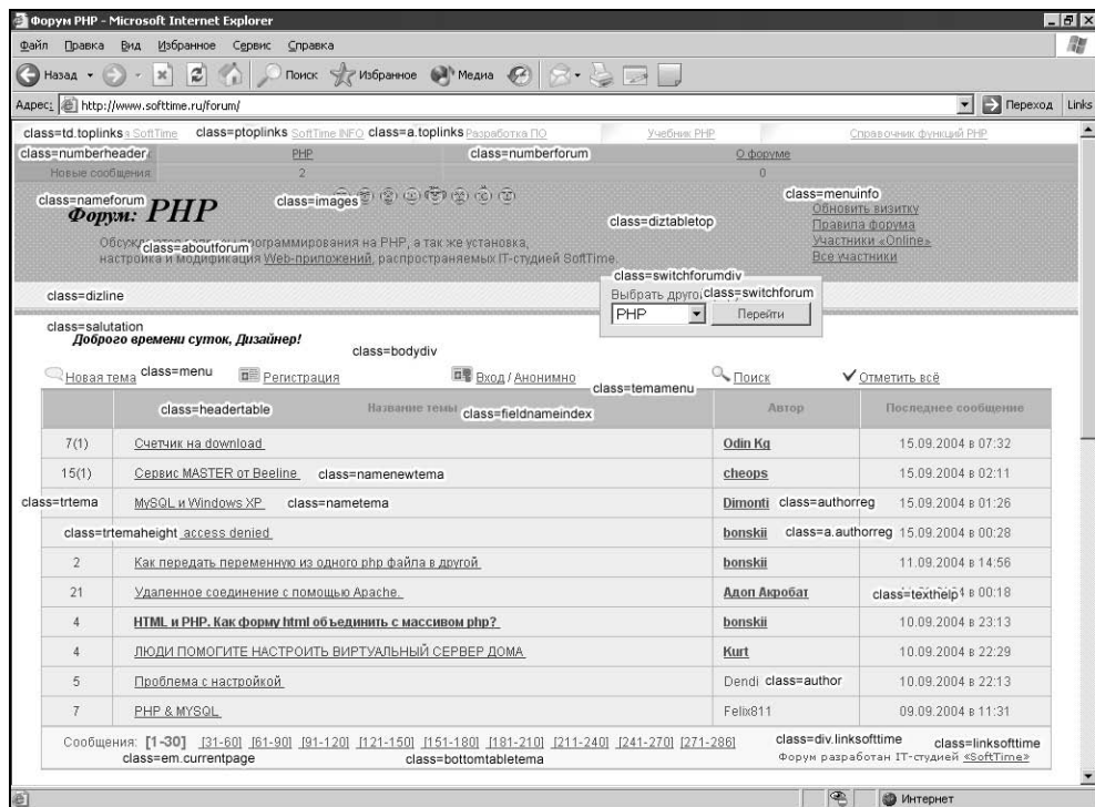
Рис. 20.10. Карта стилей для страницы index.php
