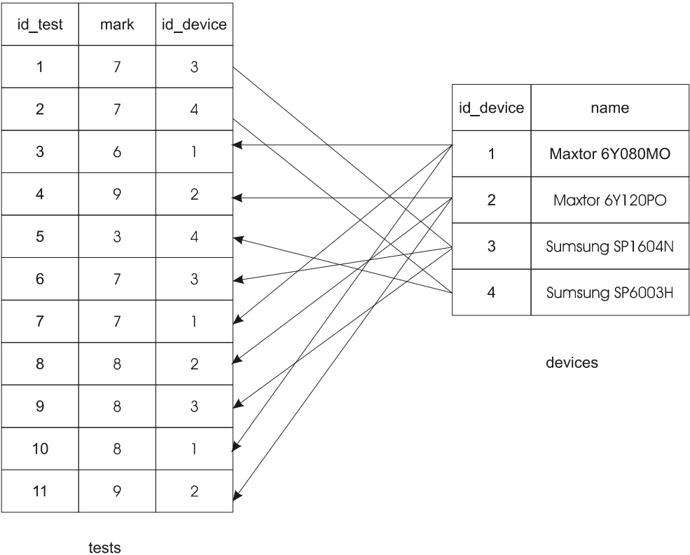
Рис. 2.25. Система оценок: таблицы tests и devices
