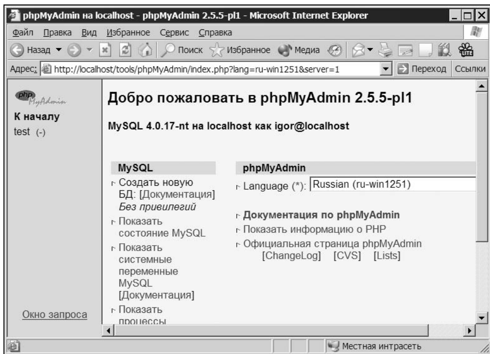
Рис. 2.31. Доступ разрешен только к одной базе данных — test, остальные базы данных не доступны
