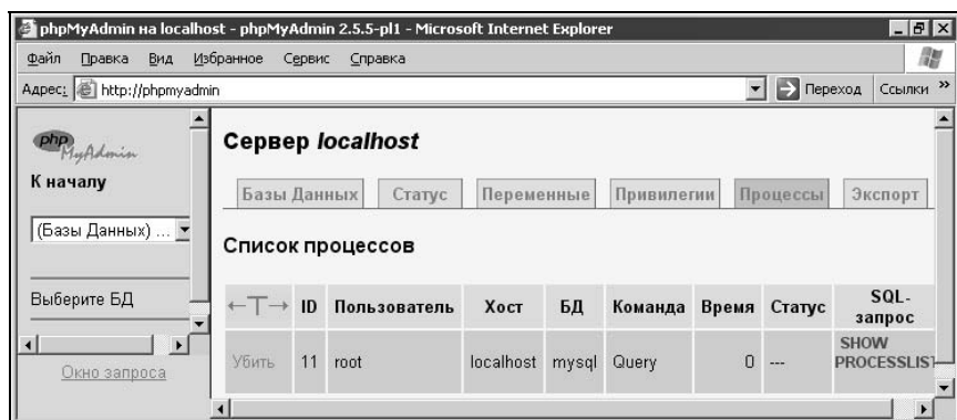
Рис. 2.38. Список процессов, запущенных на сервере MySQL
