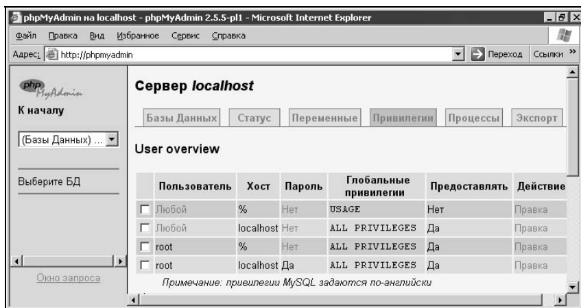
Рис. 2.39. Список пользователей сервера MySQL и их привилегий
