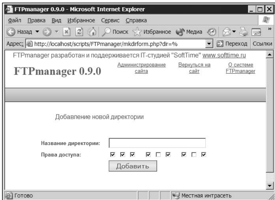
Рис. 16.2. Форма для добавления новой директории
