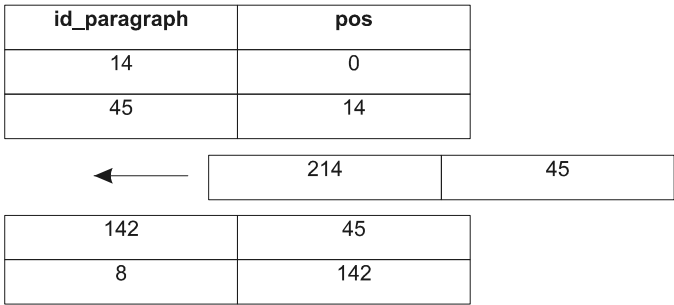
Рис. 7.15. Вставка нового параграфа со значением id_paragraph = 214
