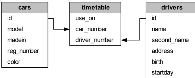
Рис. 16.2. Схема базы данных таксопарка
