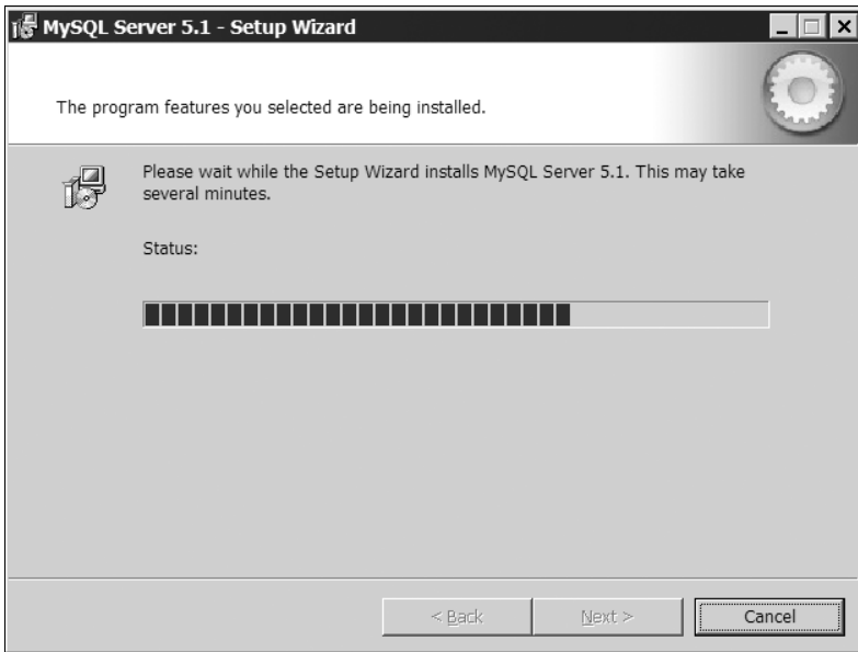
Рис. 1.24. Копирование файлов
