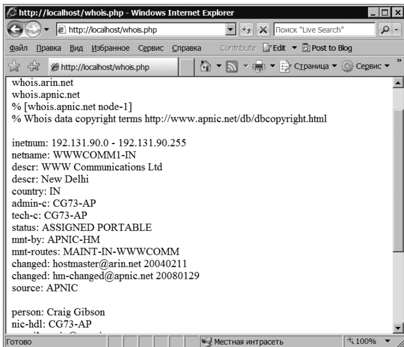
Рис. 5.9. Принадлежность IP-адреса 192.131.90.161
