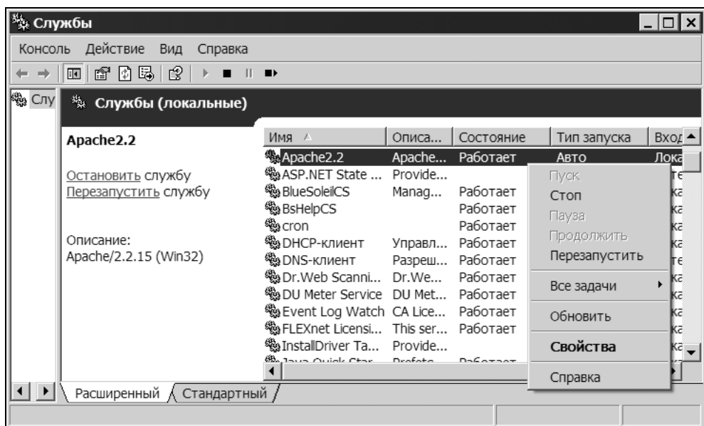
Рис. 1.10. Службы Windows
