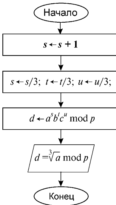
Рис. 5. Блок-схема Алгоритма 3
