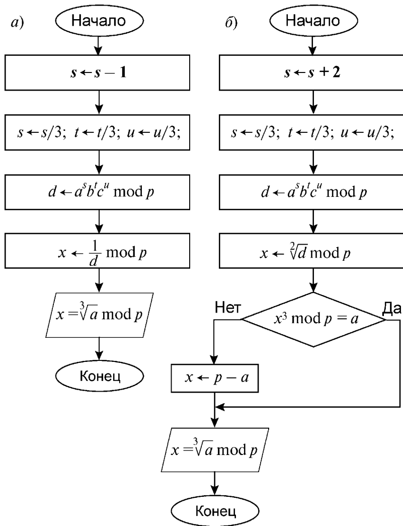
Рис. 4. Две версии Алгоритма 2: a — с вычислением обратных значений и б — с извлечением квадратного корня по модулю p
