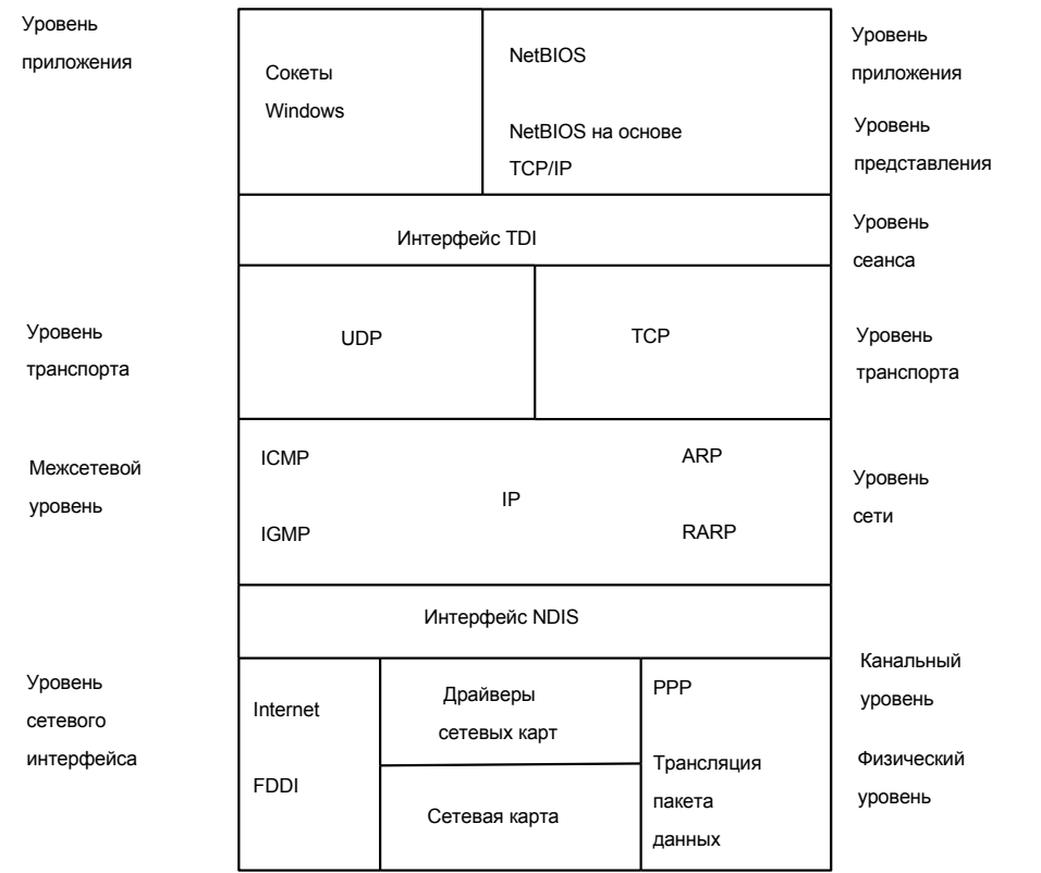
Рис. 4.1. Модель OSI и вариант от MS
