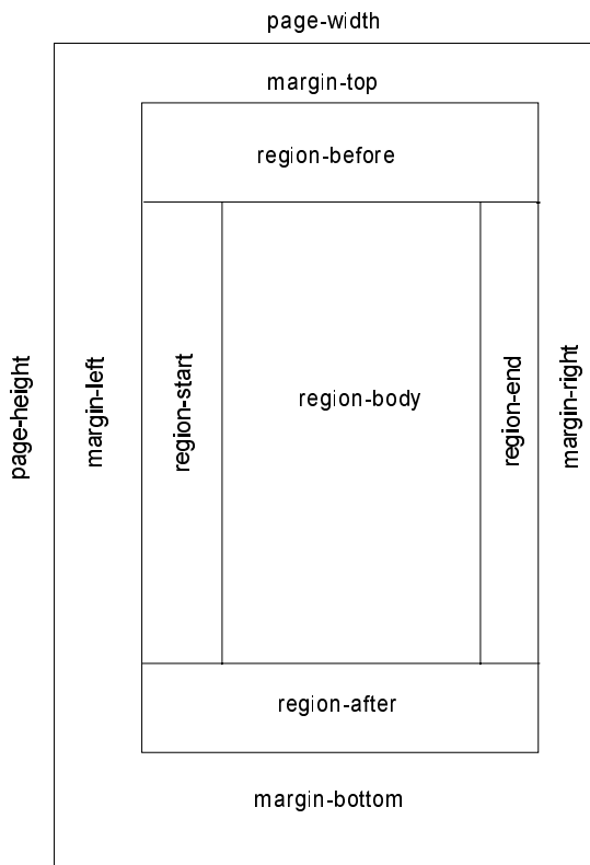
Рис. 9.1. Страница XSL
