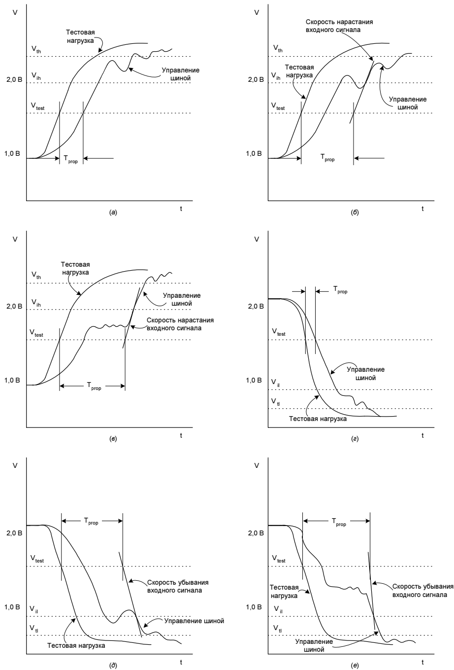
Рис. 9.4. Измерение T_{prop} для сигнальной среды 5 В
