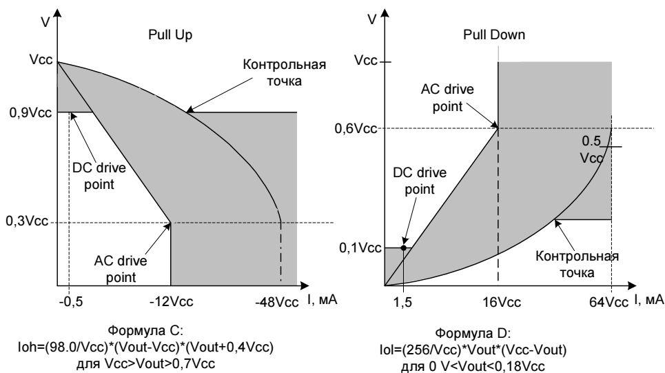
Рис. 8.4. ВАХ для сигнальной среды 3,3 В
