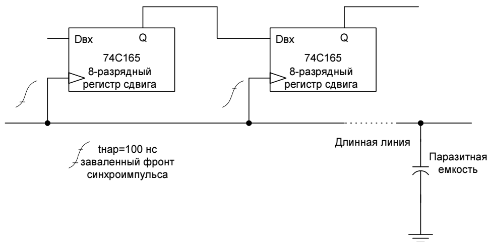
Рис. 2.6. Перекос тактовых импульсов
