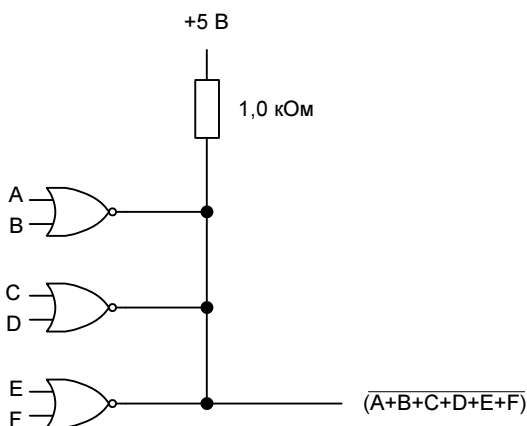
Рис. 2.4. Проводное ИЛИ
