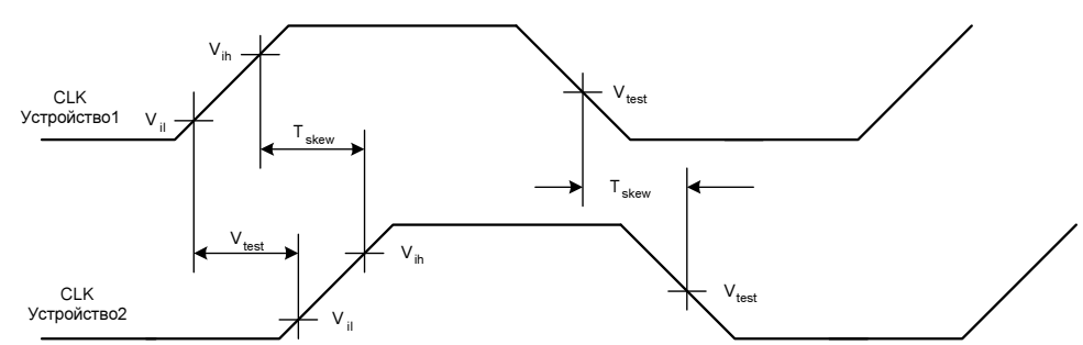
Рис. 9.1. Параметры перекоса тактовых импульсов
