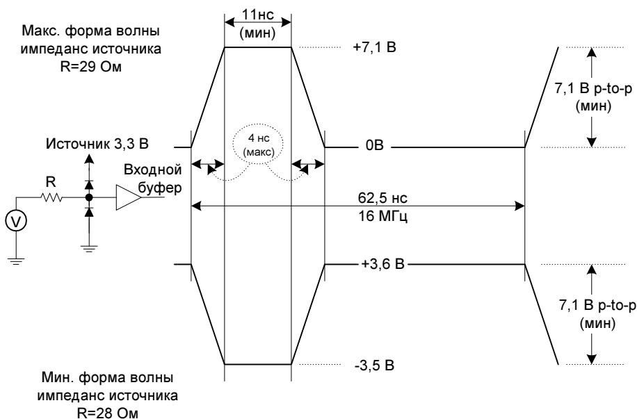
Рис. 8.6. Форма максимального сигнала для среды 3,3 В
