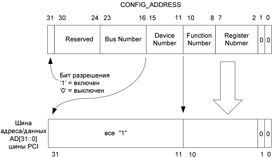
Рис. 3.7. Преобразование типа "0"
