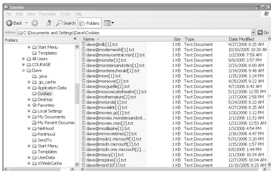
Рис. 5.4. Папка Cookies
