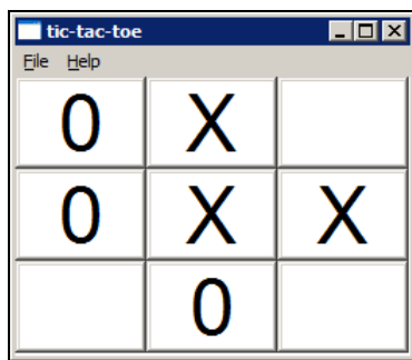
Рис. 3.1. Крестики-нолики
