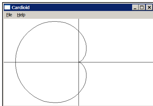
Рис. 1.13. Кардиоида
