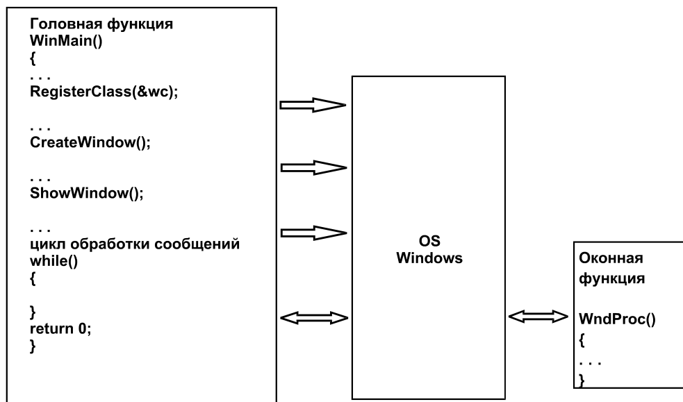
Рис. 1.1. Структура Windows-приложения
