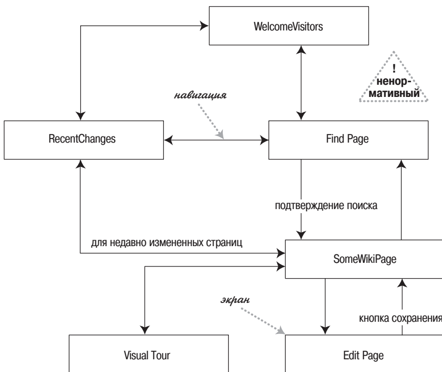
Рис. 1.3. Неформальная диаграмма потока экранов для части wiki ( http://c2.com/cgi/wiki )
