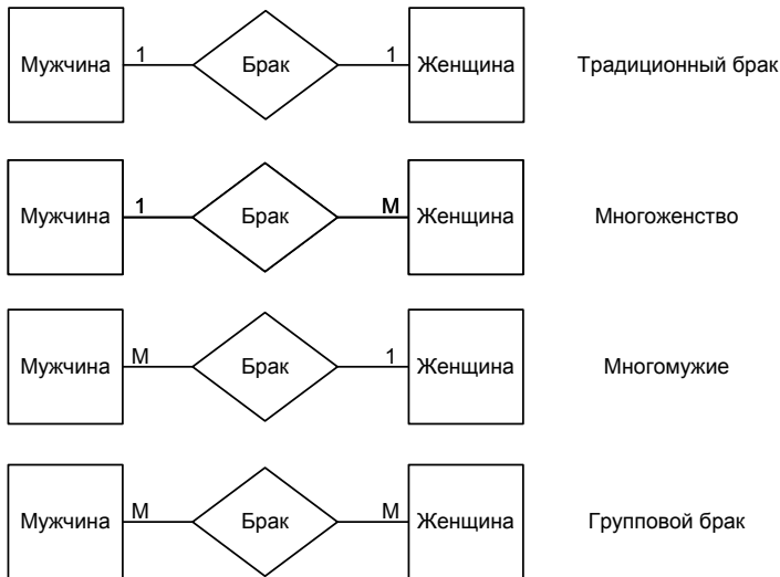
Рис. 2.3. Возможные связи между двумя сущностями
